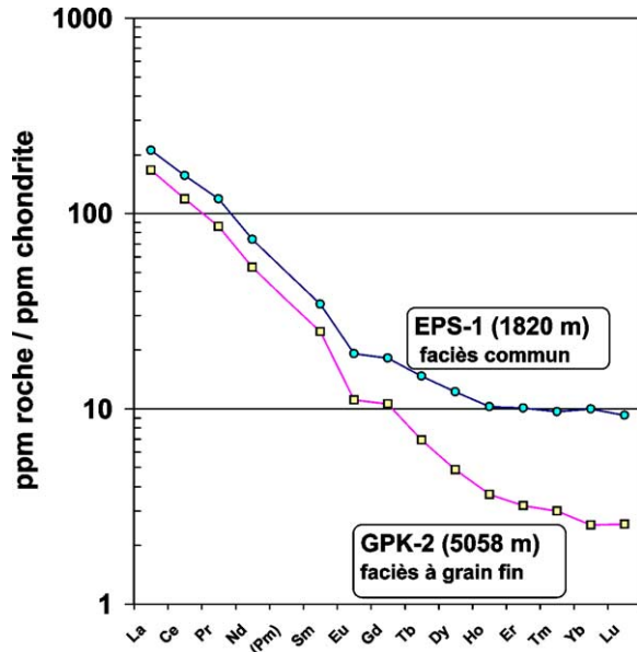
Fig. 5. Spectres de terres rares normalisés par rapport aux chondrites pour les deux granitoïdes de Soultz (valeurs de normalisation d’après les teneurs de la chondrite Leedy, divisées par 1,2, mesurées par Nakanura et Masuda [15] et Masuda [14]).
