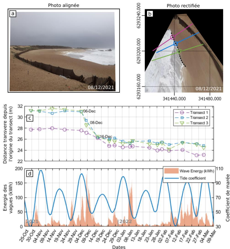
Figure 2. (a) Photo citoyenne prise à la station du Santocha le 08/12/2021 et alignée par rapport à la photo de référence de ce site (non montrée). (b) Image rectifiée et centrée sur la partie du merlon proche du poste d'observation, et crête du merlon digitalisée (courbe noire discontinue). (c) Evolution temporelle de la position transverse de la crête du merlon le long des trois transects représentés dans le panel (b). (d) Energie des vagues simulées (rouge) et marée astronomique (bleu) au large de Capbreton (source MARC IFREMER).
