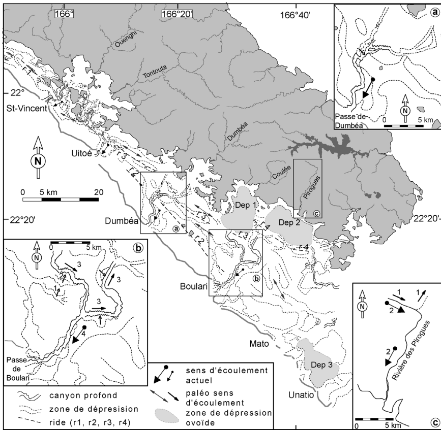
Fig. 2. Interprétation morphologique du paléoréseau hydrographique lors de l'émersion du lagon.
