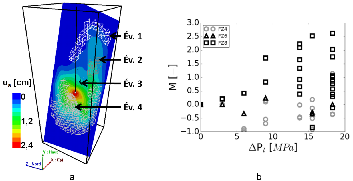
Figure 5. Magnitude des évènements microsismiques : a. illustration de l'individualisation des évènements sur FZ8 lors du dernier palier de surpression, et b. moments sismiques des évènements individualisés sur les FZ4, FZ6 et FZ8
