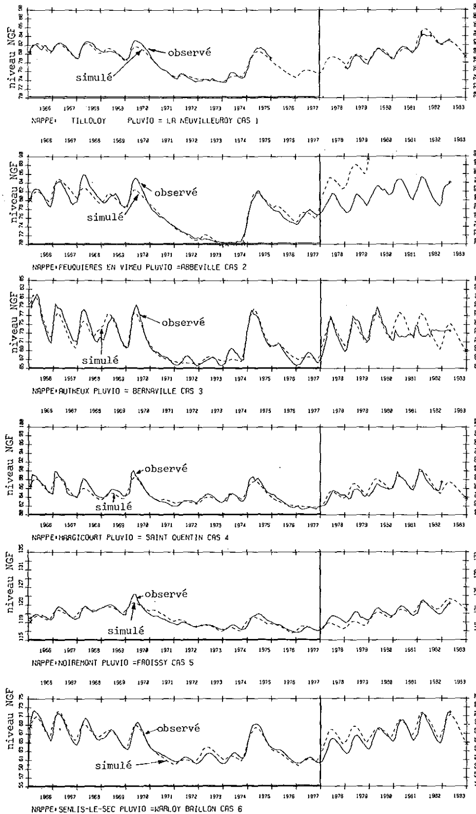
FIG. 2. — Calage de 13 piézomètres sur la période 1966-1977.
