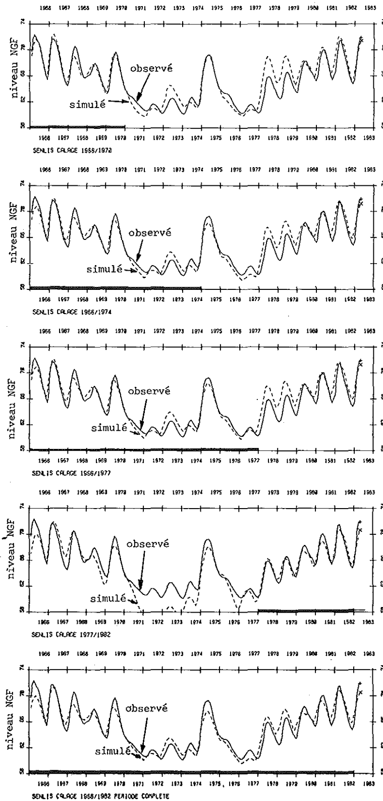
FIG. 4. — Piézomètre Senlis : calage sur 5 périodes différentes.
