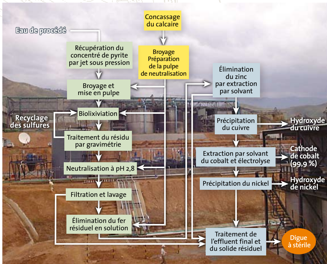
Fig. 5 : Schéma général simplifié de l'installation de production de cobalt de la Kasese Cobalt Company Ltd. (Ouganda).
