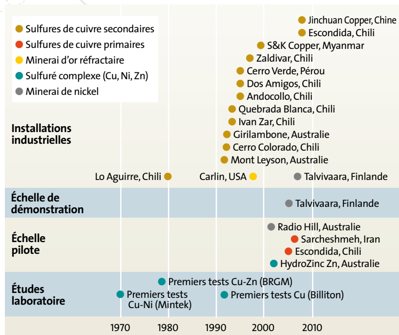
▲ Fig. 6 : Liste non-exhaustive des installations de biolixiviation en tas dans le monde.
