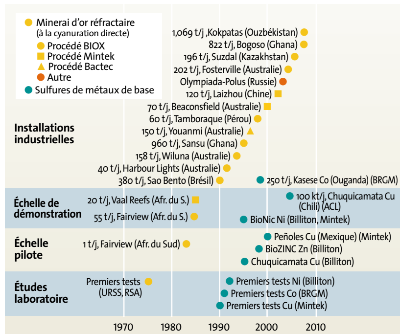
▲ Fig. 7 : Liste non-exhaustive des installations de biolixiviation en cuve agitée dans le monde.
