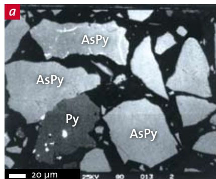
Fig. 2 : Libération de grains d'or piégés dans de l'arséno-pyrite par biolixiviation ménagée. Photographies prises au microscope électronique à balayage. a) Avant biolixiviation, en électrons rétrodiffusés. b) Après un traitement par biolixiviation partiel, en électrons secondaires pour montrer la corrosion de l'arséno-pyrite à l'endroit des fractures du minéral sulfuré.
